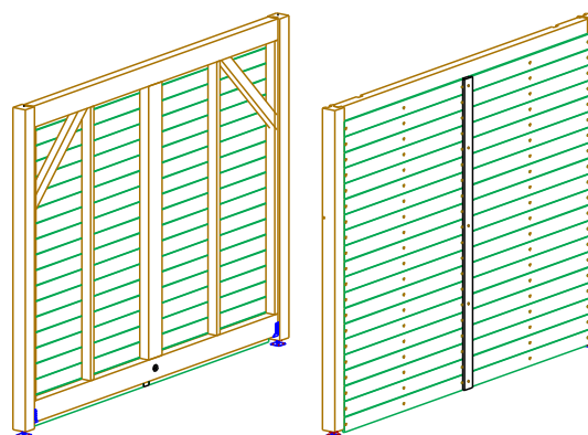
Bardage horizontal Modèle ouvert ou semi ouvert
