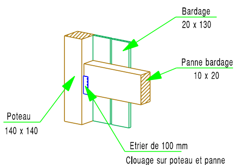
Détail Sabot Métallique
