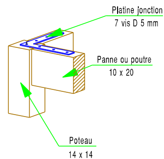
Détail Platine de Jonction
