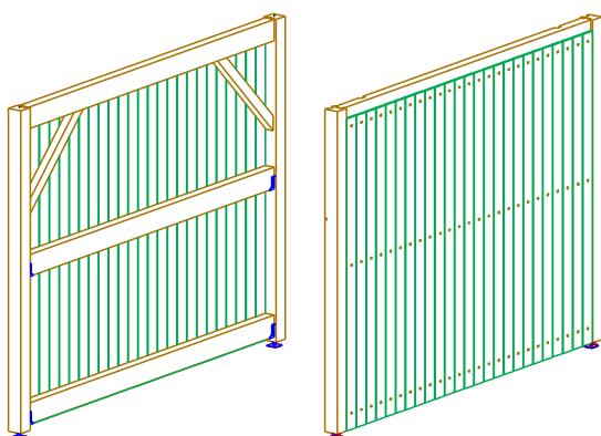
Bardage vertical Modèle ouvert ou semi ouvert
