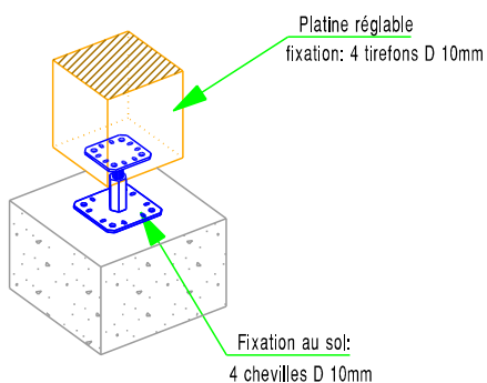
Détail Pied de Poteau
