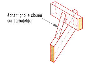
Fixation panne sur arbalétrier
